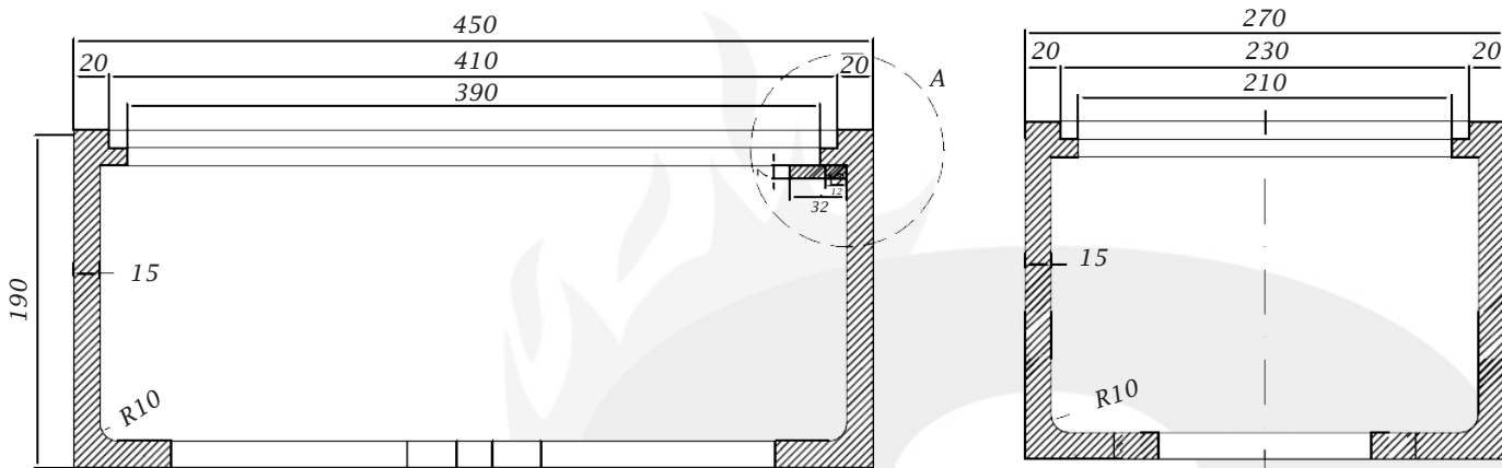
SECCIÓN A-A
