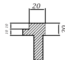
SECCIÓN C-C
