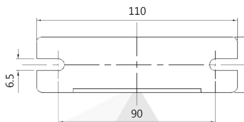
Soporte de montaje Externo (modelo S). Material: Acero inoxidable AISI 316.
