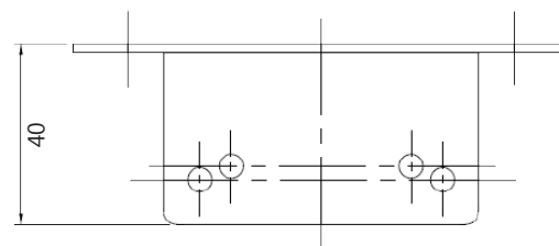
Soporte de montaje Externo (modelo S). Material: Acero inoxidable AISI 316.
