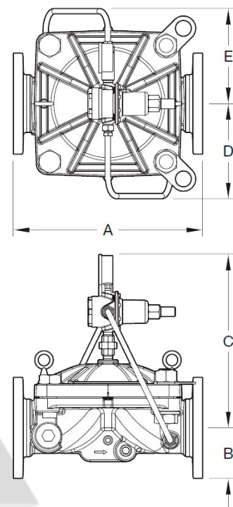
Figura 9: Válvula PRV-1A: Conexiones finales Brida x Brida - Medidas nominales de la instalación.
