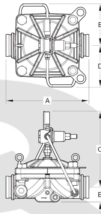
Figura 8: Válvula PRV-1A: Conexiones finales Ranura x Ranura - Medidas nominales de la instalación.
