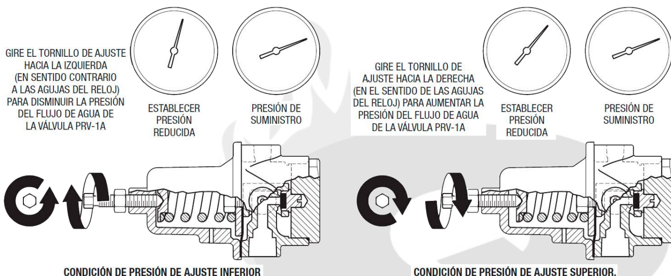
Figura 5: Válvula reductora de presión modelo PRV-1A: montaje y ajuste de la válvula piloto modelo P1.
