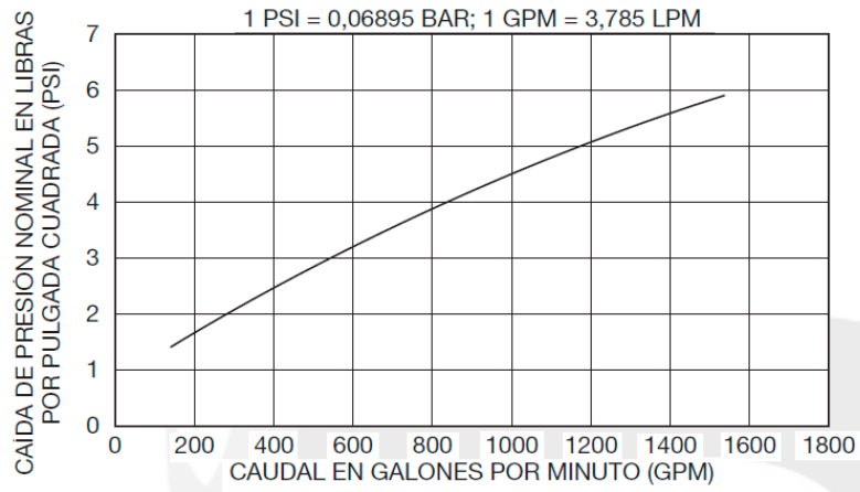
Gráfico D: Válvula reductora de presión PRV-1A de 6" (DN150) - Caída mínima de presión.
