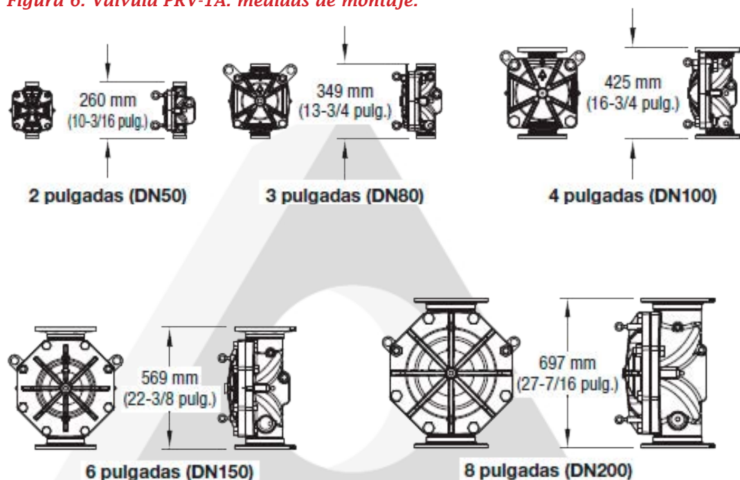
Figura 6: Válvula PRV-1A: medidas de montaje.
