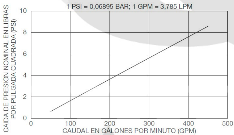
Gráfico B: Válvula reductora de presión PRV-1A de 3" (DN80) - Caída mínima de presión.
