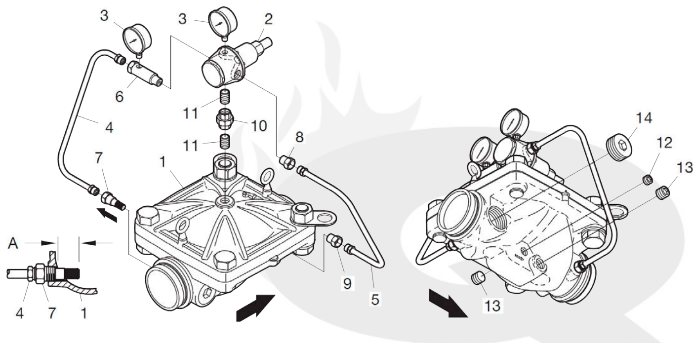
Figura 7: Válvula reductora de presión modelo PRV-1A: conjunto de parte de accesorios (trim)
