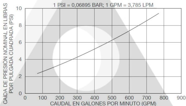
Gráfico C: Válvula reductora de presión PRV-1A de 4" (DN100) - Caída mínima de presión.
