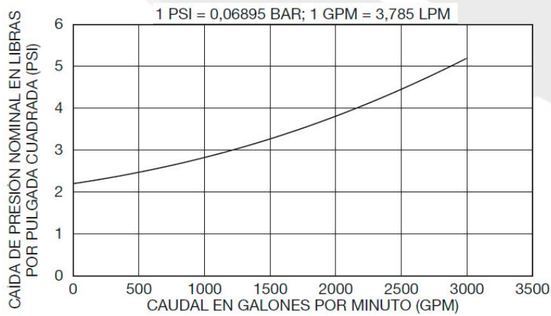
Gráfico E: Válvula reductora de presión PRV-1A de 8" (DN200) - Caída mínima de presión.
