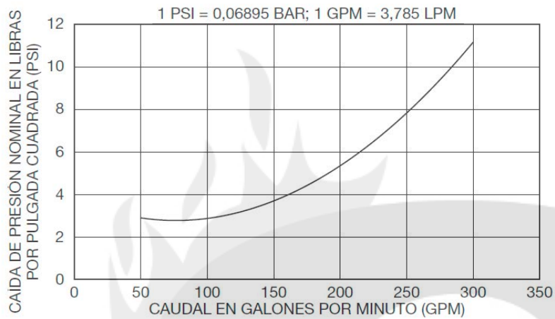
Gráfico A: Válvula reductora de presión PRV-1A de 2" (DN50) - Caída mínima de presión.
