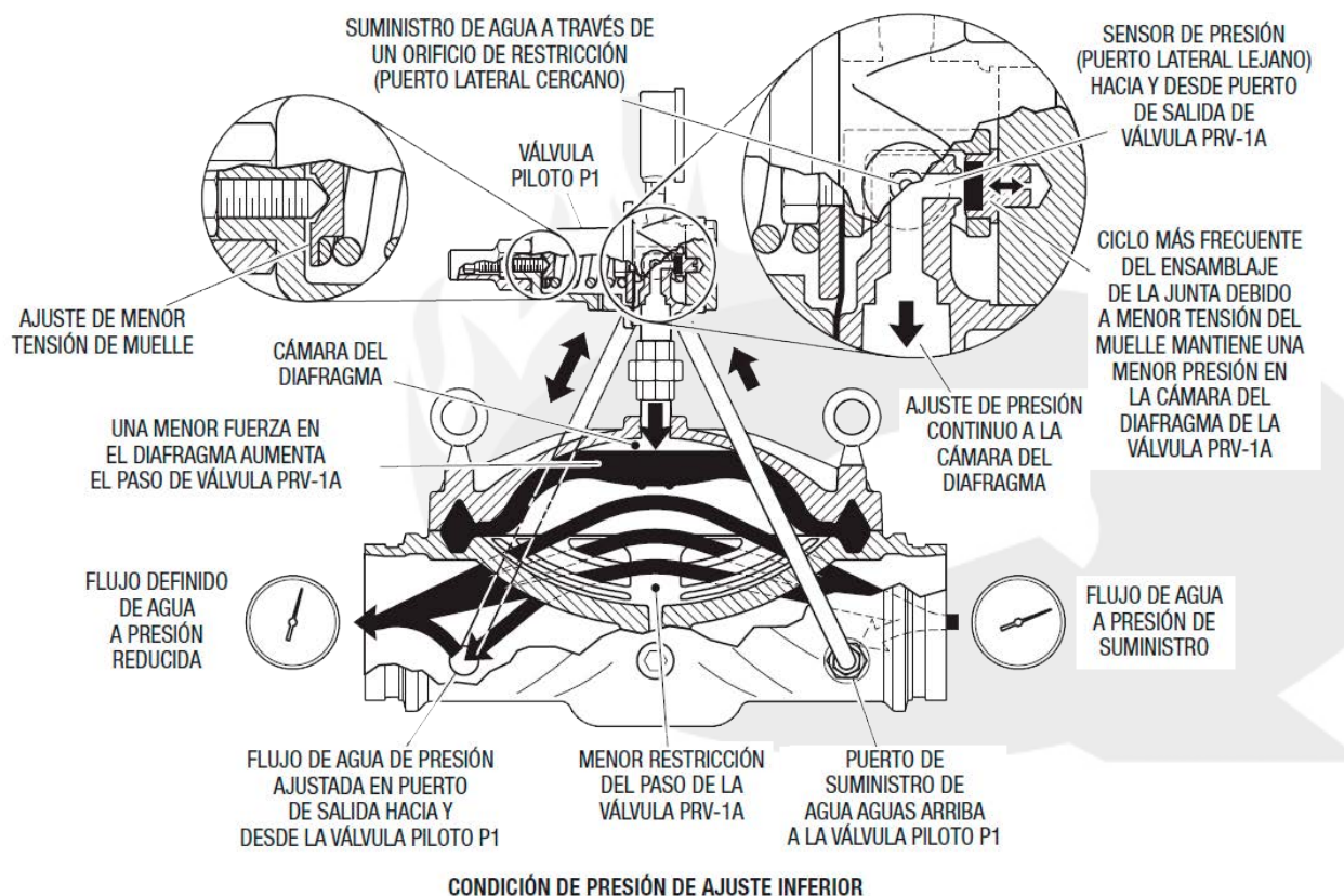
Figura 4: Válvula reductora de presión modelo PRV-1A: funcionamiento.
