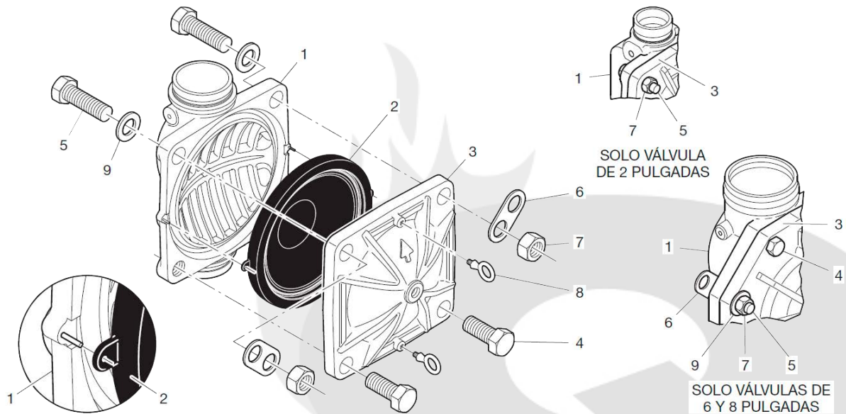
Figura 3: Conjunto de válvula DV-5A.
