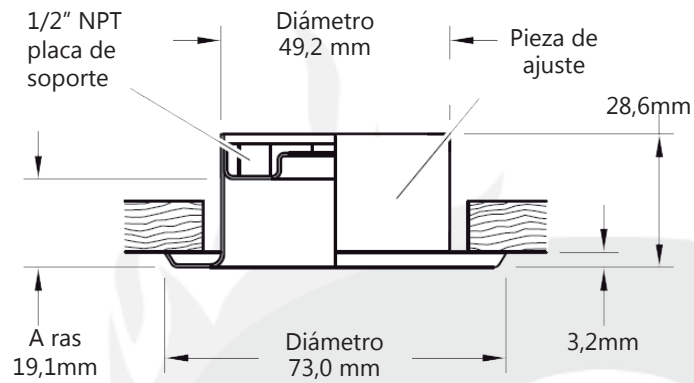
Figura 1 - Estilo 10: 1/2" NPT con ajuste de 19,1mm.
