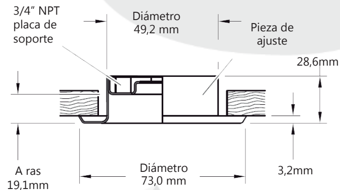
Figura 2 - Estilo 40: 3/4" NPT con ajuste de 19,1mm.
