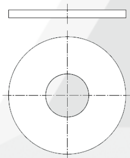
Arandela ala ancha cincada DIN 9021
