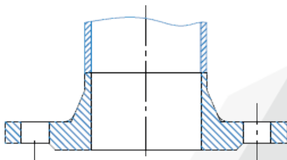
BRIDA CUELLO
