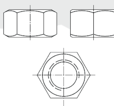
Varilla roscada cincada DIN 975 (clase 4.8)
