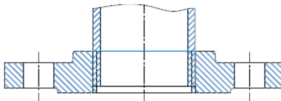
BRIDA CUELLO ROSCADA
