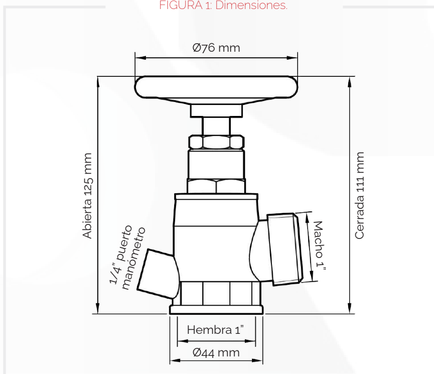
FIGURA 1: Dimensiones.
