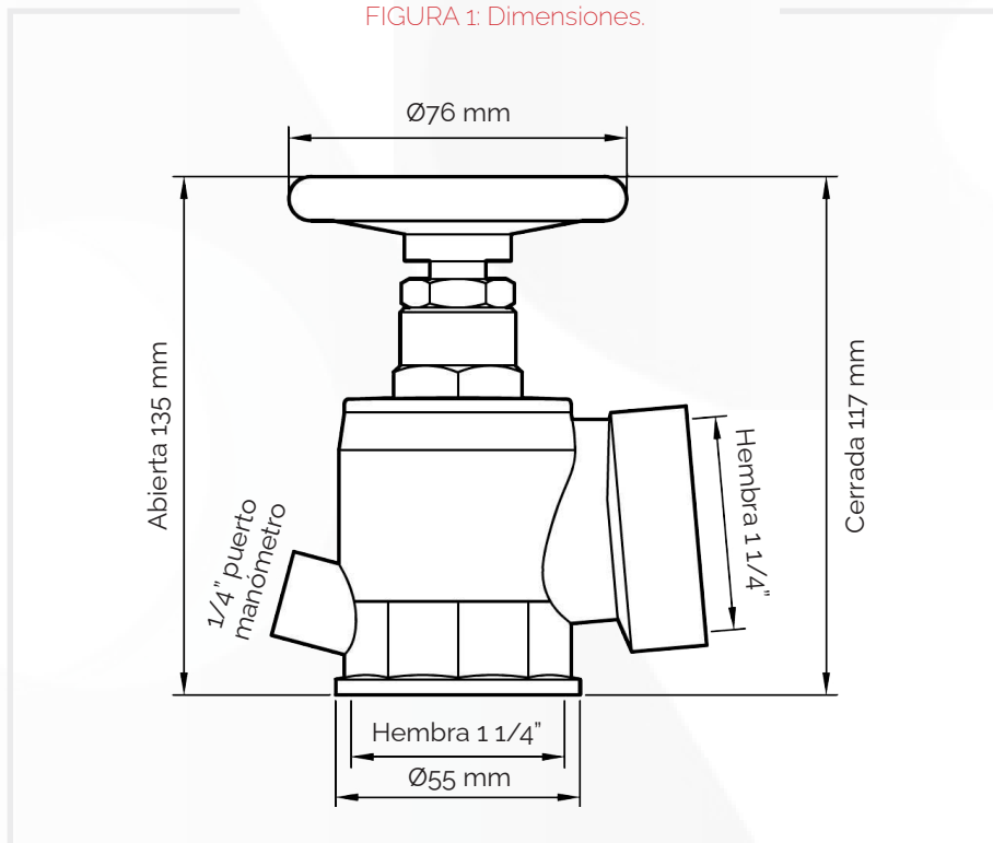
FIGURA 1: Dimensiones.
