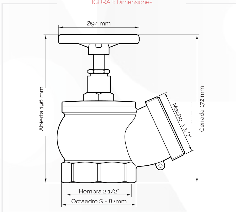
FIGURA 1: Dimensiones.
