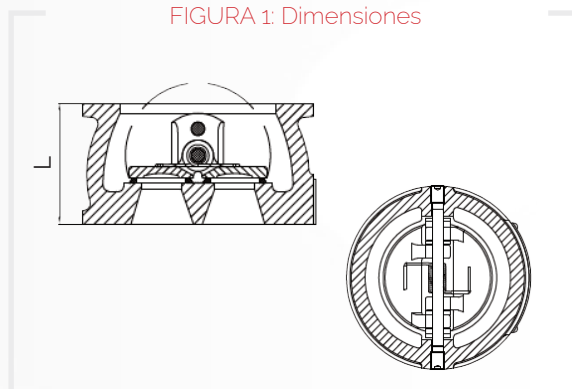
FIGURA 1: Dimensiones
