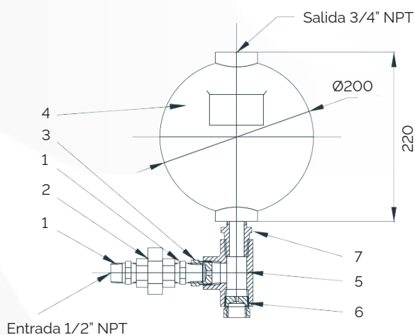
FIGURA 1: Dimensiones y componentes
