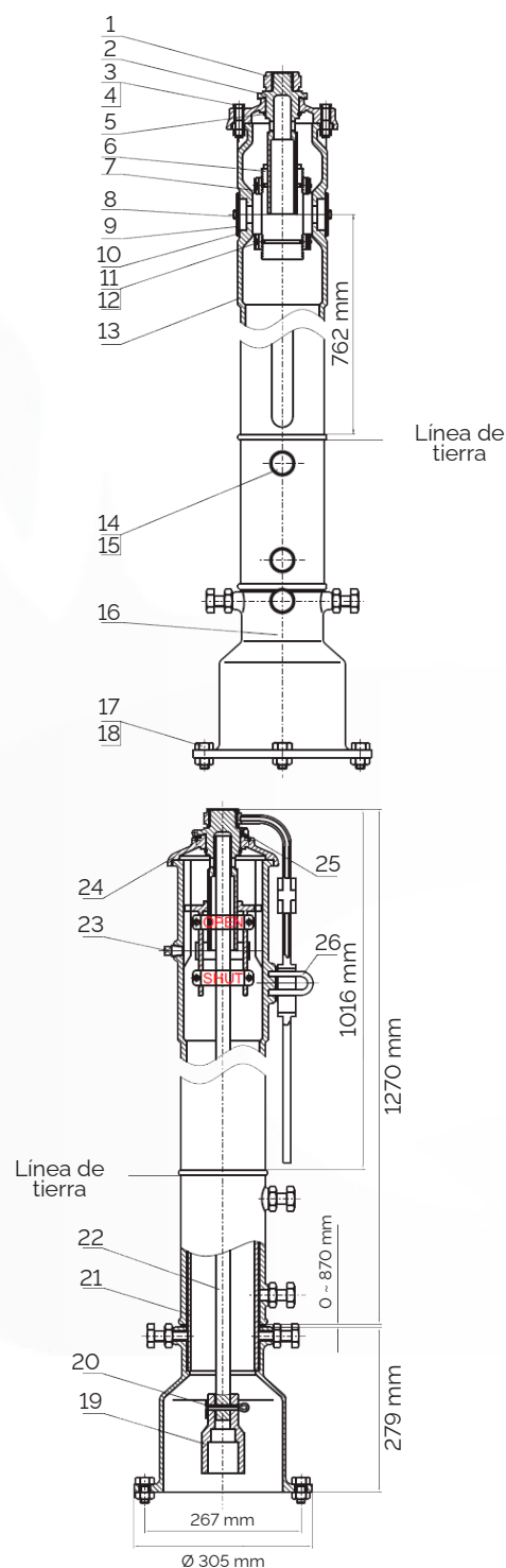
FIGURA 1: Dimensiones
