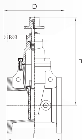
FIGURA 1: Dimensiones
