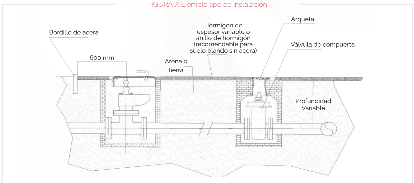
FIGURA 7: Ejemplo tipo de instalación
