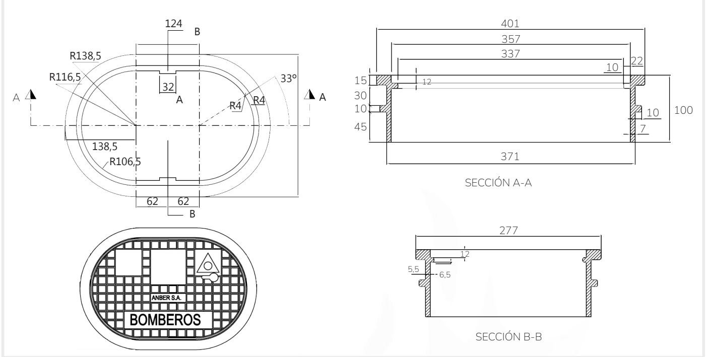
FIGURA 4: Plano Arqueta para GEYSER 1 BOCA
