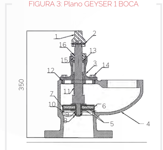
FIGURA 3: Plano GEYSER 1 BOCA
