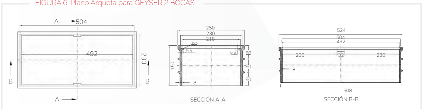
FIGURA 6: Plano Arqueta para GEYSER 2 BOCAS
