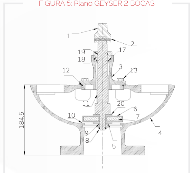
FIGURA 5: Plano GEYSER 2 BOCAS
