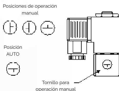
Figura 5: Esquema solenoide (16)
