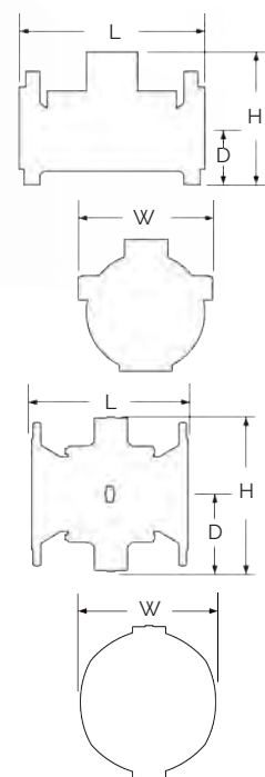
Figura 3: Plano conexión embreada.
