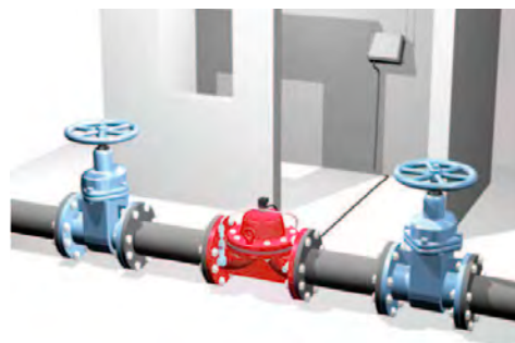
Válvula con solenoide de Dorot, controlada por un controlador local.
