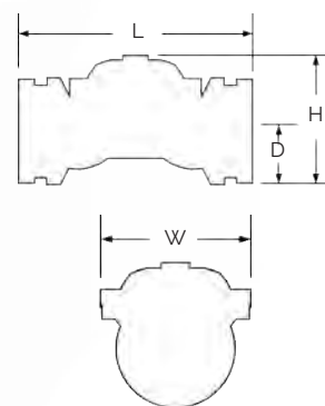
Figura 3: Plano conexión embreada.
