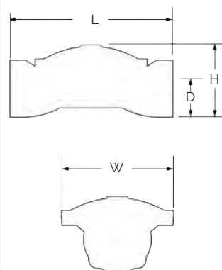
Figura 2: Plano conexión ranurada.
