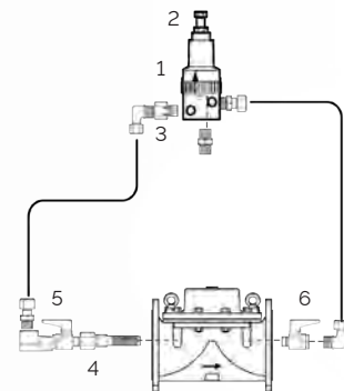
Figura 4: Componentes del sistema de control
