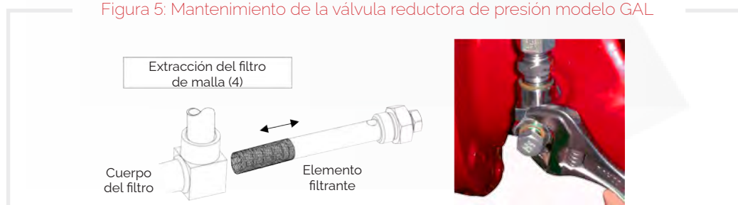
Figura 5: Mantenimiento de la válvula reductora de presión modelo GAL
