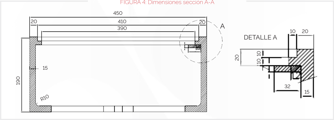
FIGURA 4: Dimensiones sección A-A
