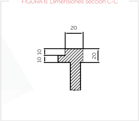
FIGURA 6: Dimensiones sección C-C
