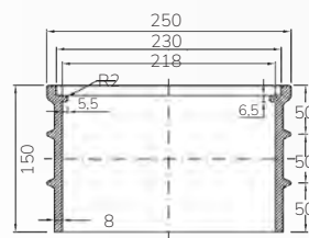
SECCIÓN A-A
