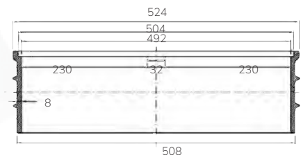
SECCIÓN B-B
