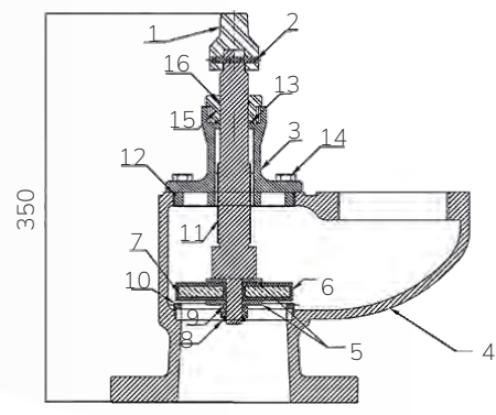
FIGURA 3: Plano GEYSER 1 BOCA
