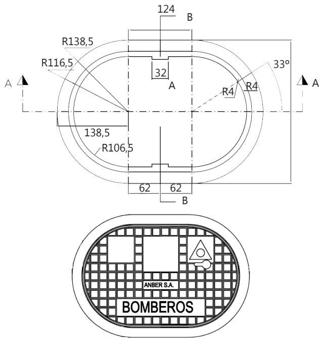
FIGURA 4: Plano Arqueta para GEYSER 1 BOCA
