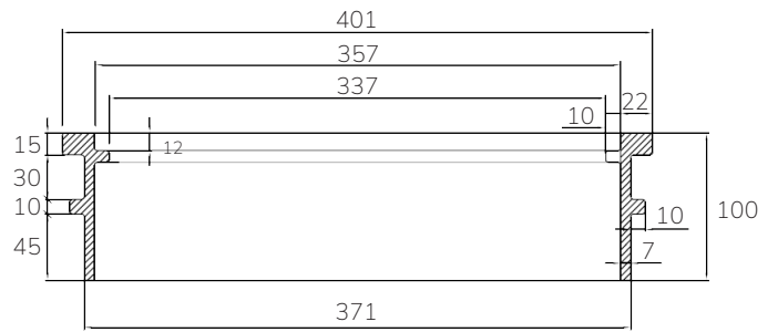
SECCIÓN A-A
