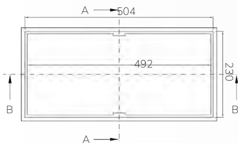
FIGURA 6: Plano Arqueta para GEYSER 2 BOCAS
