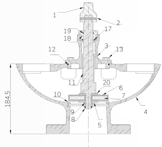
FIGURA 5: Plano GEYSER 2 BOCAS
