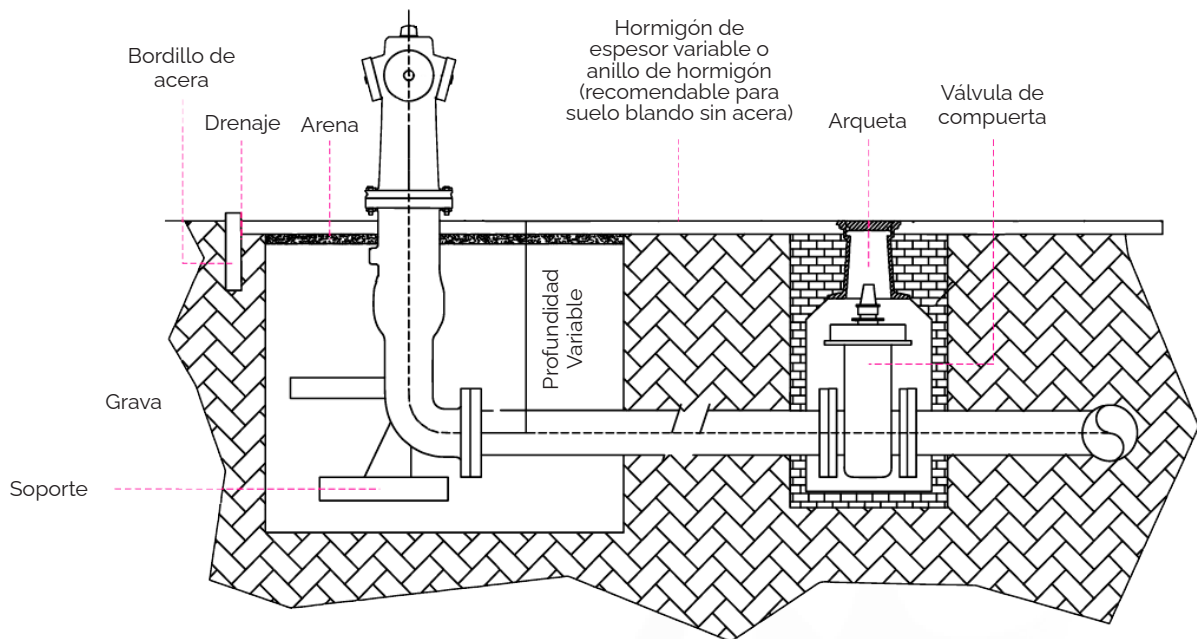
FIGURA 12: Ejemplo tipo de instalación
